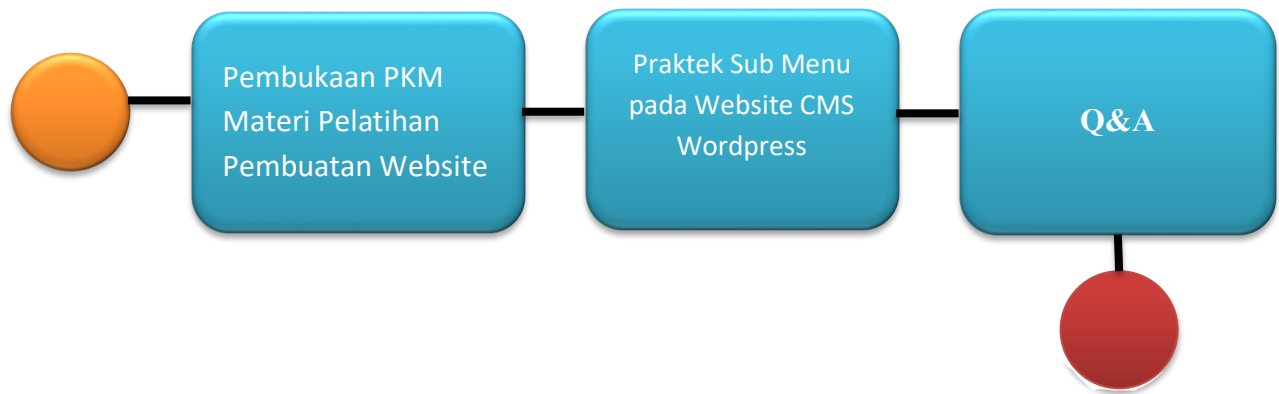
Gambar 1. Diagram Aktivitas
