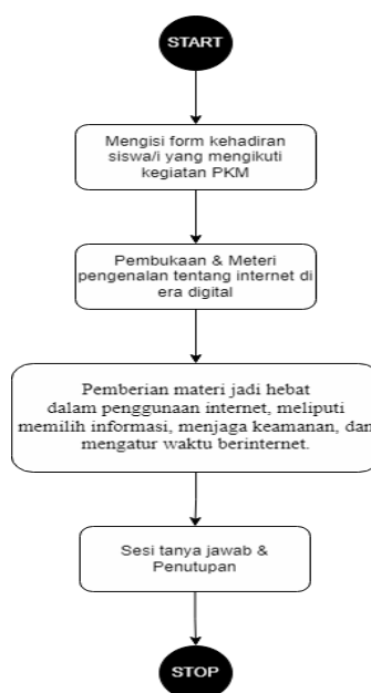
Gambar 1. Diagram Aktivitas
